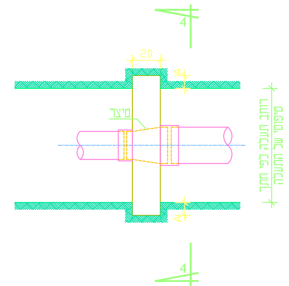
תכנית מסי 4
