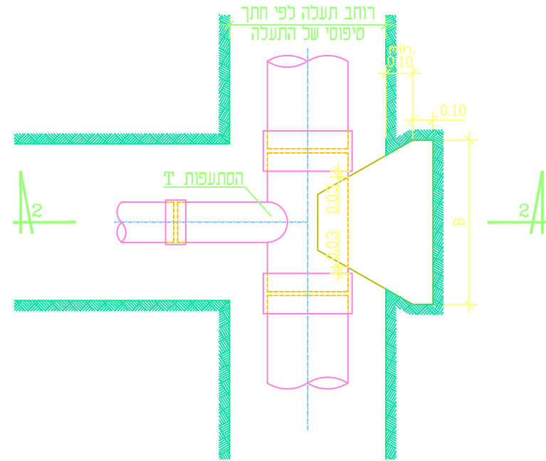
תכנית מסי 2
