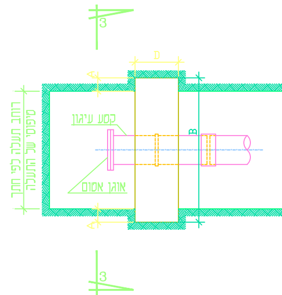
תכנית מסי 3
