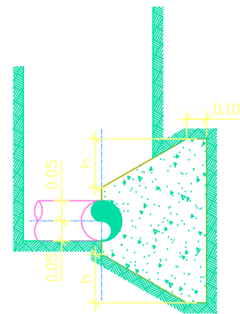
חיתוך 1-1
